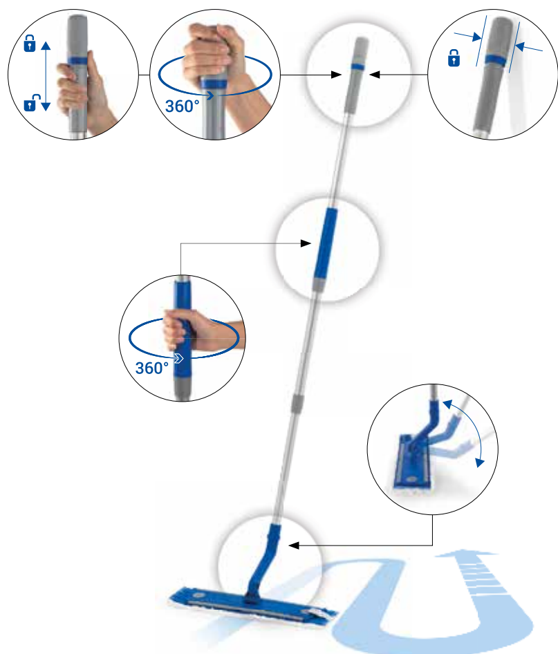
La rotazione dell'impugnatura superiore può essere bloccata per appoggiare ErgoSwing in sicurezza.
