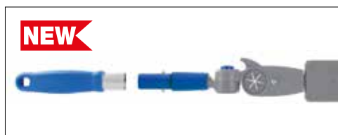
Versione con foro: -per aste telescopiche -per manici telescopici e manici in alluminio a 3 fori, con l'aggiunta del cono cod. P179041A
