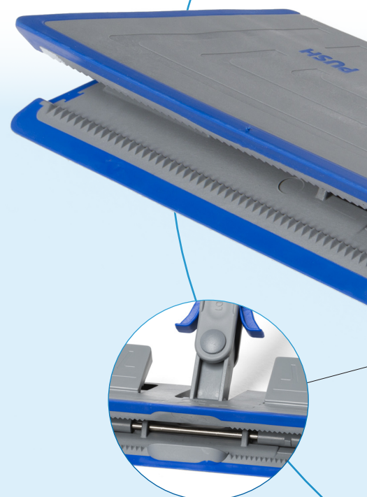
Sistema di aggancio con rilievo centrale e dentatura
